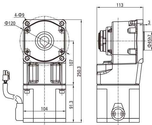
输出轴内孔结构
