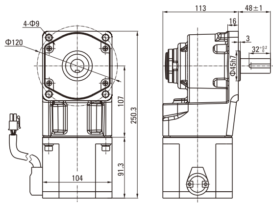
输出轴结构
